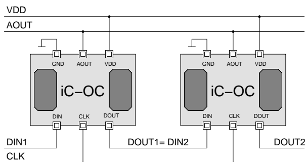
Bild 5: Beispiel Kettenschaltung für zwei Bausteine
