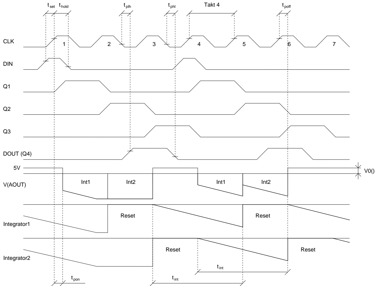
Bild 4: Zeitverhalten nach dem Einschalten (Annahme: V_0()1 = V_0()2 = V_0() , V_{DD} = 5\text{ V} )
