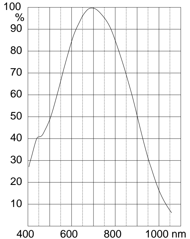
Bild 2: Relative Spektrale Empfindlichkeit im BMST
