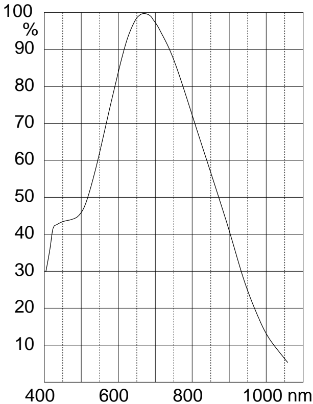
Bild 1: Relative Spektrale Empfindlichkeit
