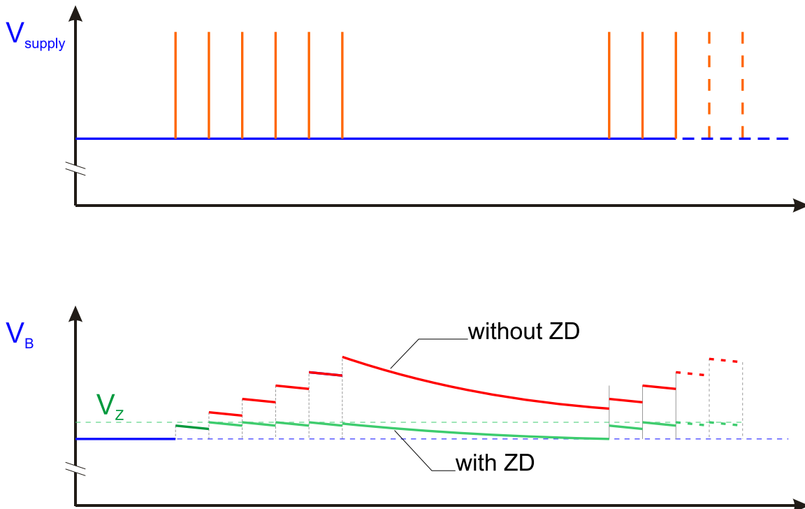
Bild 4: Spannungsbegrenzung der Versorgungsspannung mit Zenerdiode ZD
